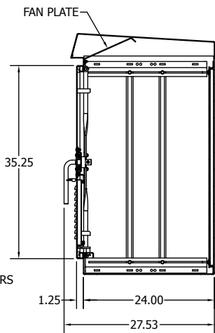
SECTION D-D
